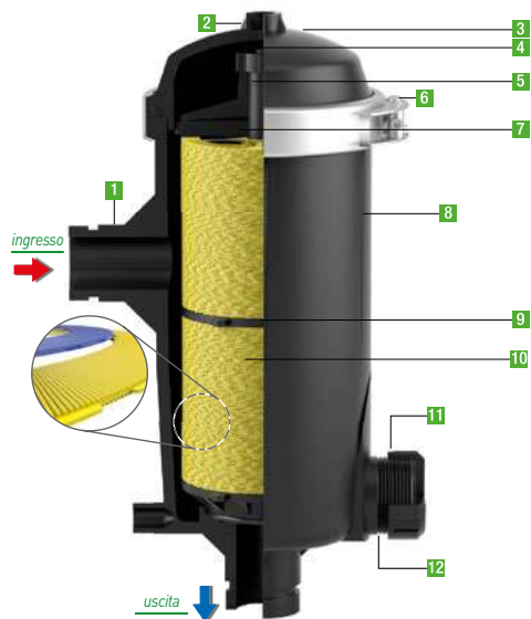
FILTRO A DISCHI
