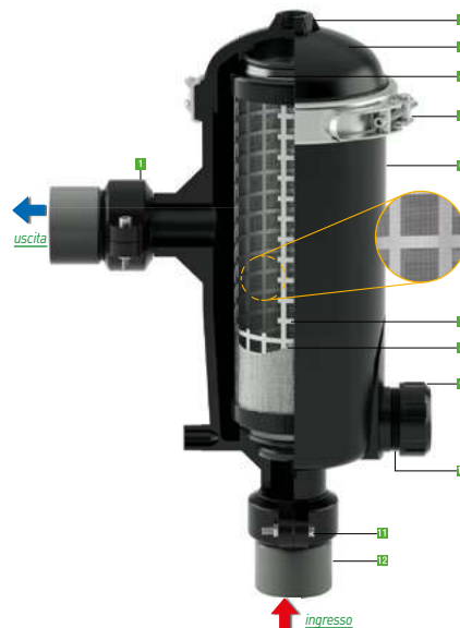
FILTRO A MAGLIA
